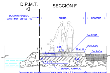
PLANO DE SECCIÓN DE LA ACERA MARÍTIMA
